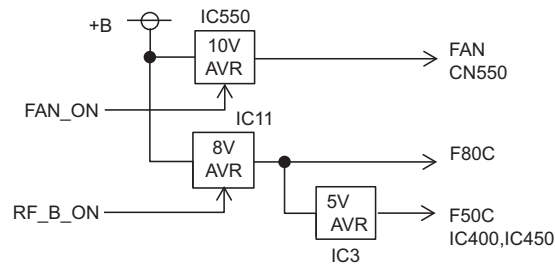
Fig.10 AVR circuit
