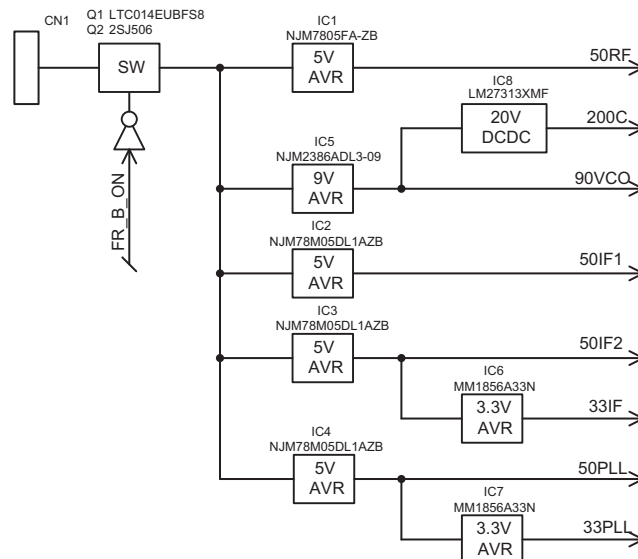
Fig.16 AVR circuit
