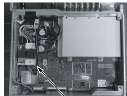
KAP-2 cable
